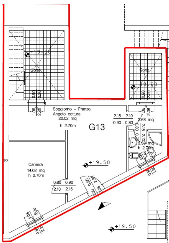
Zona soggiorno/cucina
